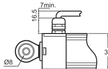
Cable output (optional)
